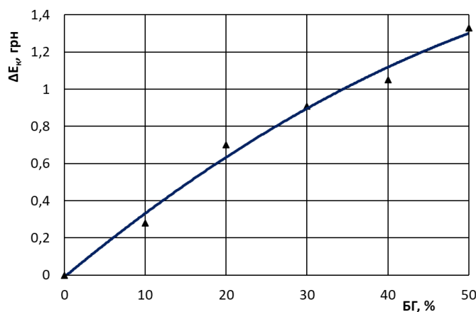
Рисунок 1 – Залежність ефективності застосування еквівалентних палив на базі СПГ від відсоткового вмісту в них біогазу
