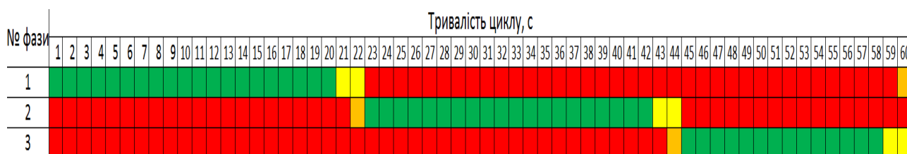
Рисунок 1 – Координовані цикли світлофорного регулювання для перехрестя Прспект Миру – вул. Набережна, зсув дорівнює 0 секунд
