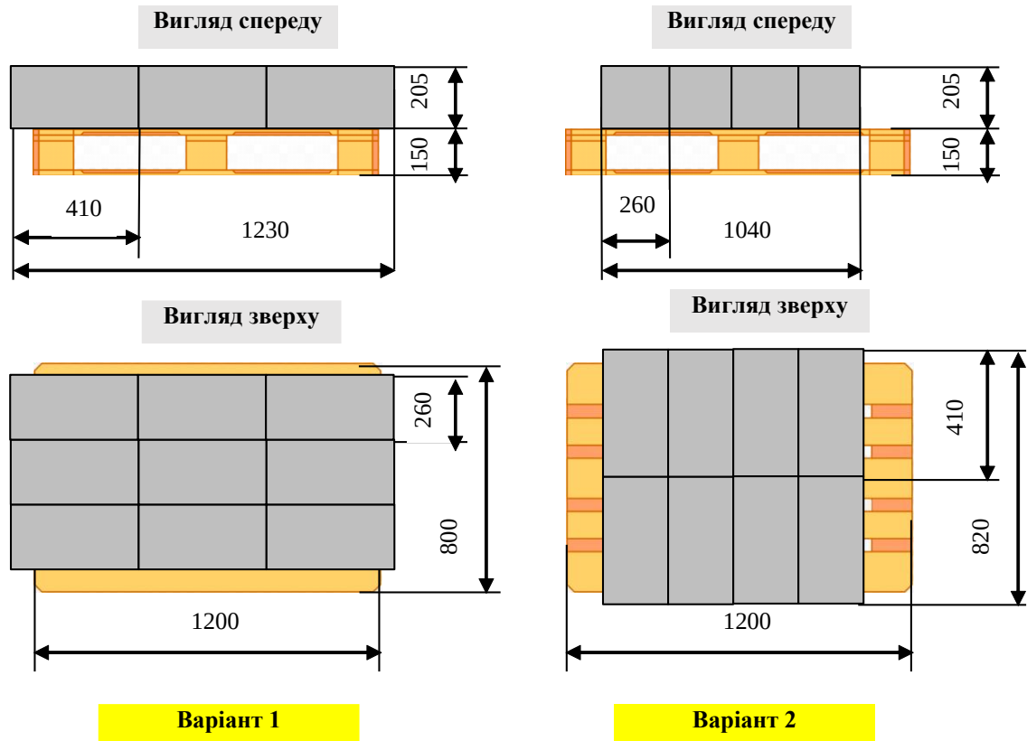
Рисунок 2 – Схема розміщення ящиків в один ярус на піддоні: варіант 1 – 9 ящиків, варіант 2 – 8 ящиків
