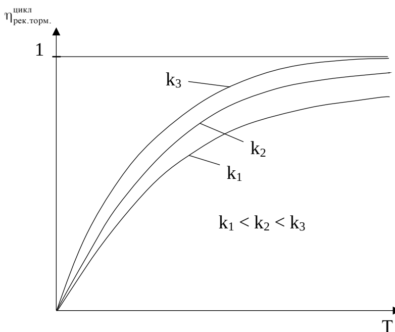
Рисунок 1 - Зависимость \eta_{\text{рек.торм.цикл}} от t
