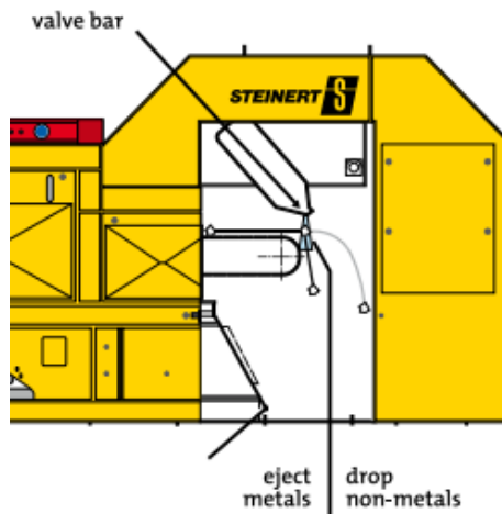
Рисунок 2 – Схема роботи індукційного сепаратора фірми Steinert (Німеччина) [2]
