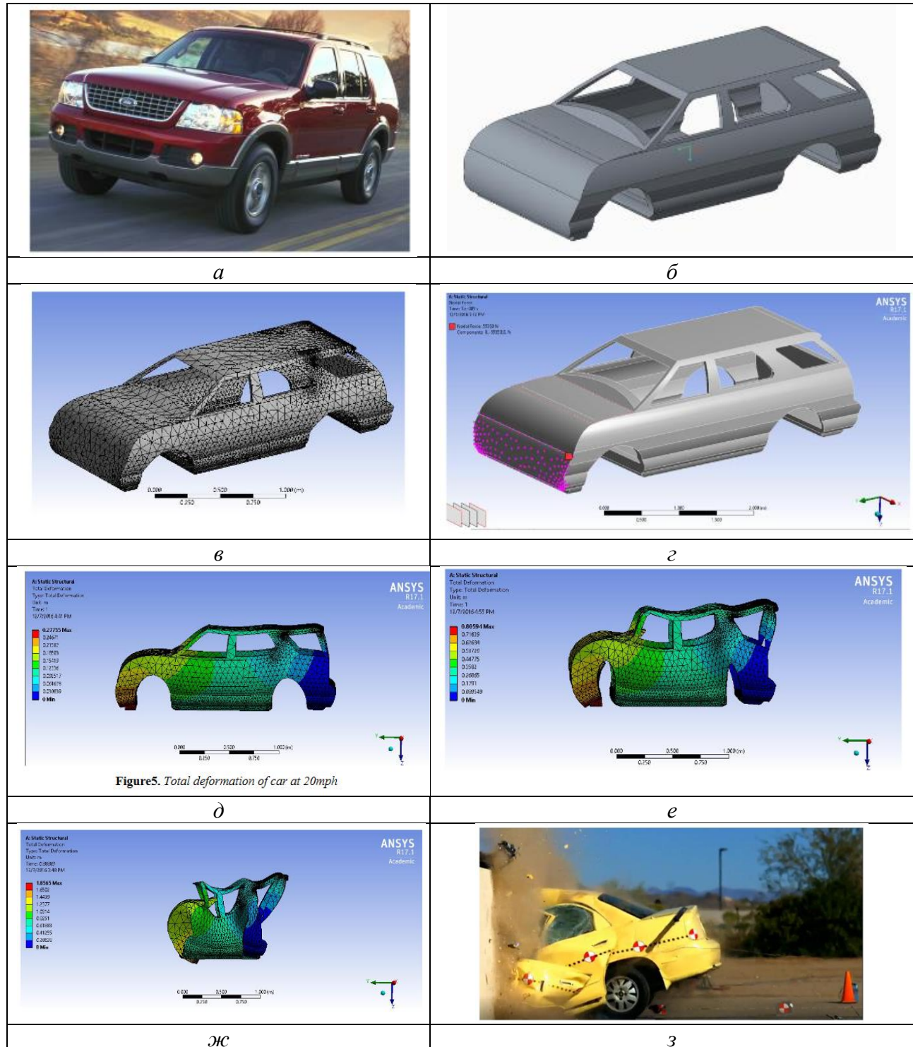
Рисунок 2 – Ізометричний вигляд Ford Explorer 2002 року ( a ). Ізометричний вигляд змодельований в CREO ( б ). Генерація сіток в ANSYS ( в ). Прикладені вузлові сили до точок контакту автомобіля ( г ). Повна деформація автомобіля на швидкості: 20 миль/год ( д ), 60 миль/год ( е ) 100 км/год ( ж ). Деформація автомобіля зі швидкістю 100 миль/год при ударі, перевірена Myth Busters ( з ).
