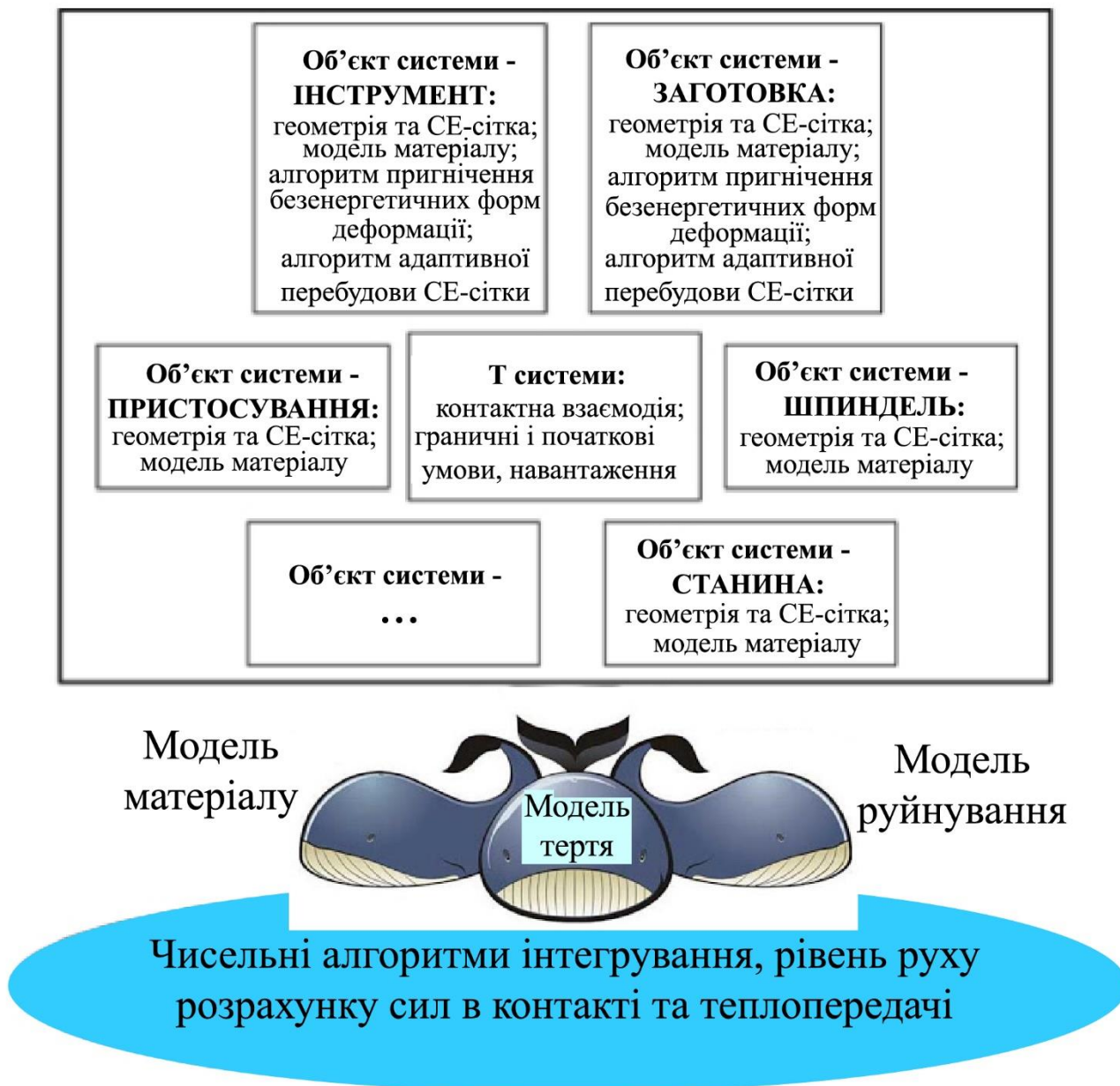
Рисунок 5 – Умовна узагальнена схема моделі процесу різання [8]
