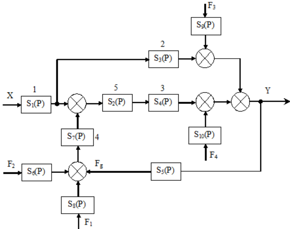
Рисунок 2 – Структурна схема регулювання гальмівних сил в гальмівній системі наведений на рисунку 1 відповідно.
