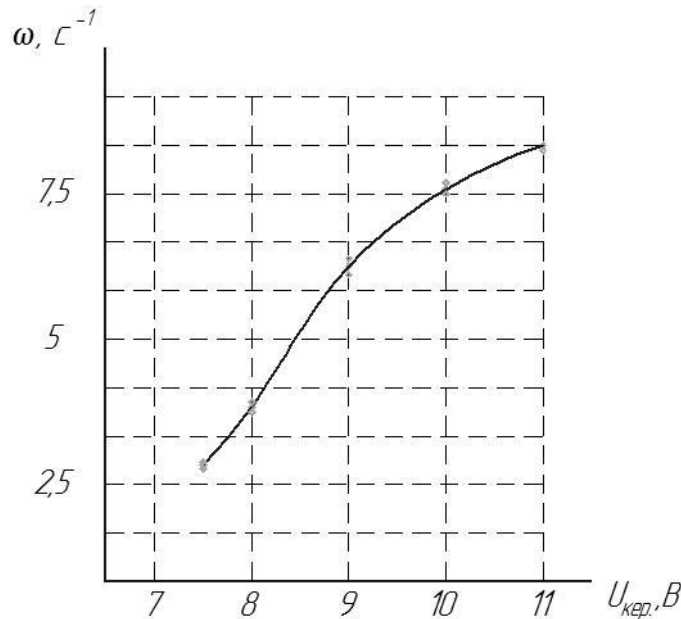
Рисунок 6 – Залежність частоти обертання гідромотора від величини напруги керування U_{\text{кер}} пропорційного електромагніта
