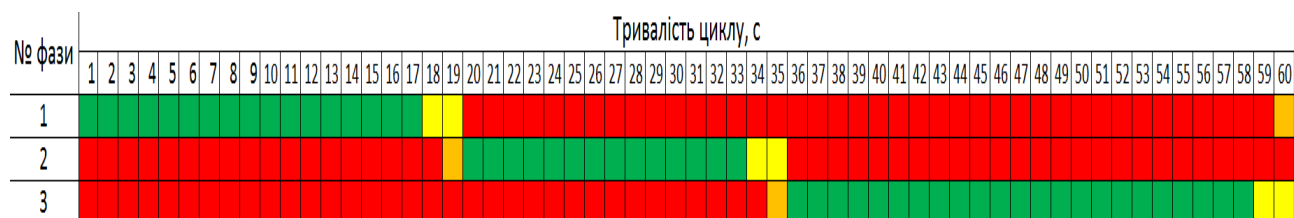
Рисунок 4 – Координовані цикли світлофорного регулювання для перехрестя Проспект Миру – вул. Міцкевича, зсув дорівнює 41 секунда
