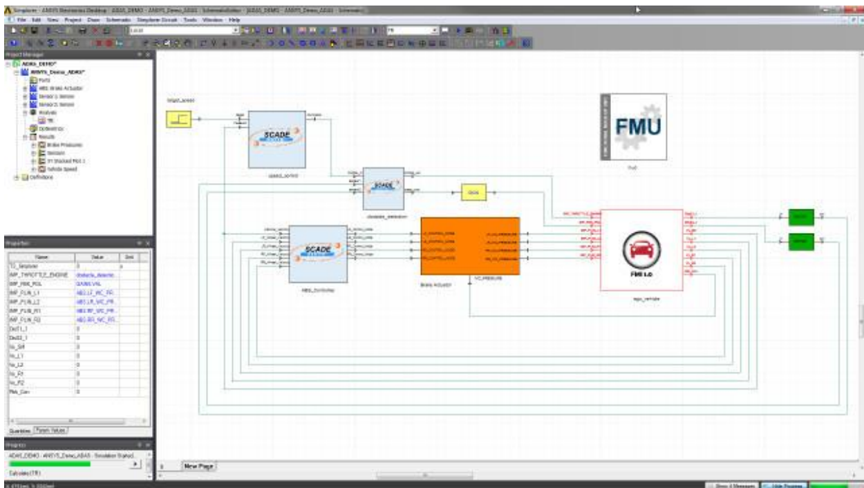
Рисунок 5 – Системна модель автопілотованого автомобіля ANSYS Simpler
